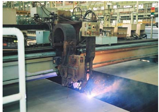
写真-6 NCプラズマ切断機
