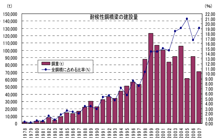
図-5 耐候性鋼橋梁の適用実績推移
