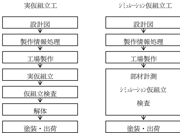
図-4 仮組立工法別による工程比較
