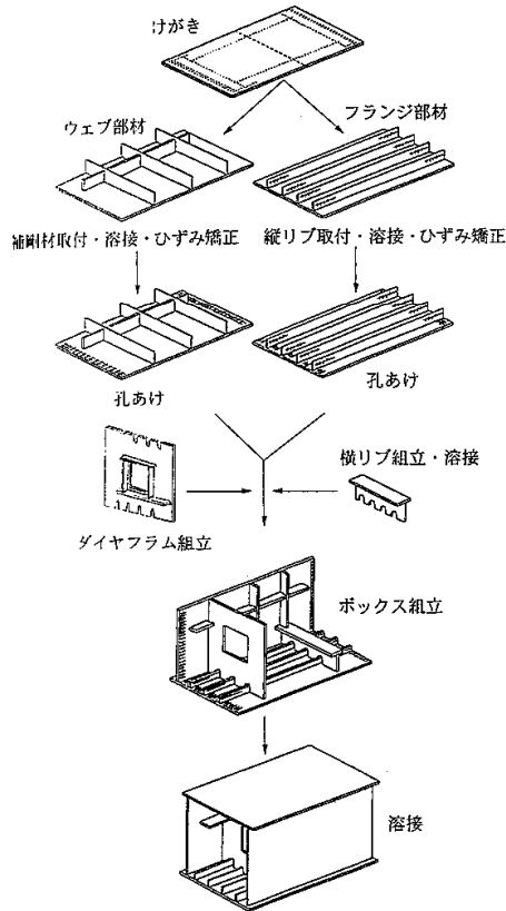
図-3 箱桁パネル工法フロー図
