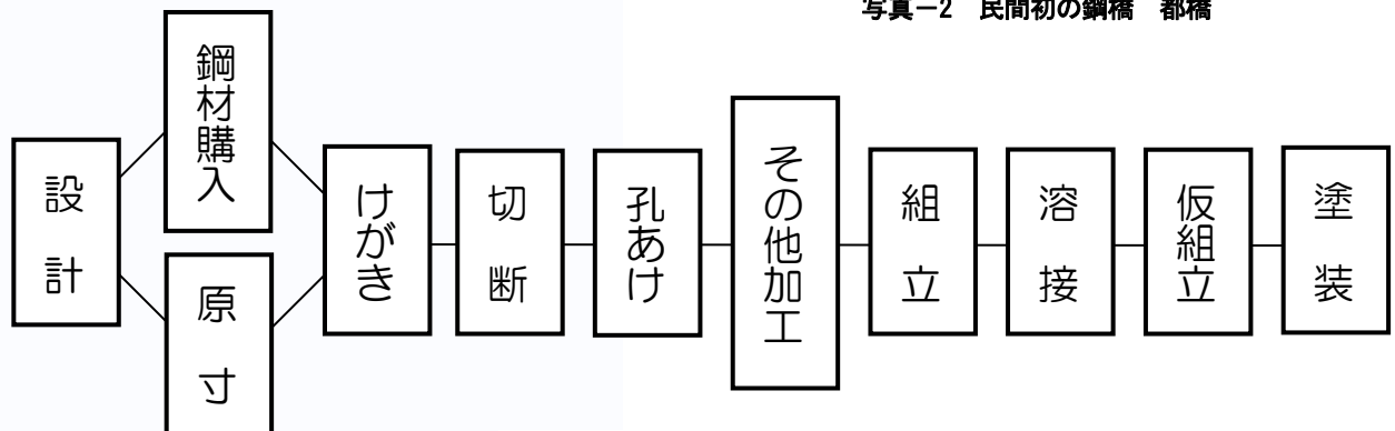
図-1 鋼橋工場製作の流れ
